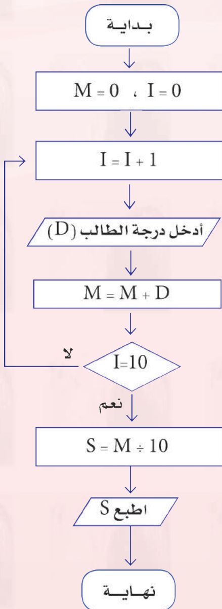
شكل (٧-٦): مخطط انسياب لحساب متوسط درجات الطلاب
